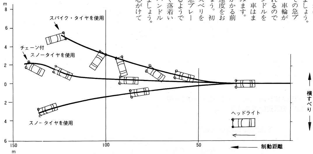
2000ccの乗用車が時速65.5km/hで直進中に急ブレーキをかけた場合（氷上）
