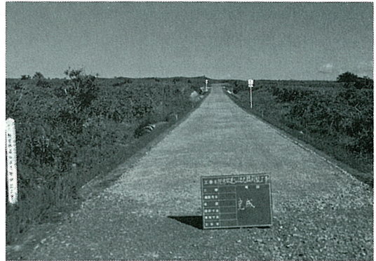
経営林道仙法志線開設工事 62年 8 月 19日完成
