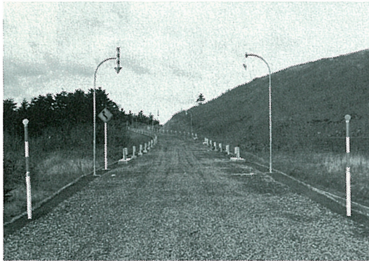
沓形線道路改良工事 62年11月30日完成
